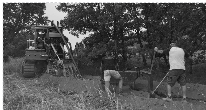
Tranchée pour ouvrir le terrain et enfouir la canalisation
